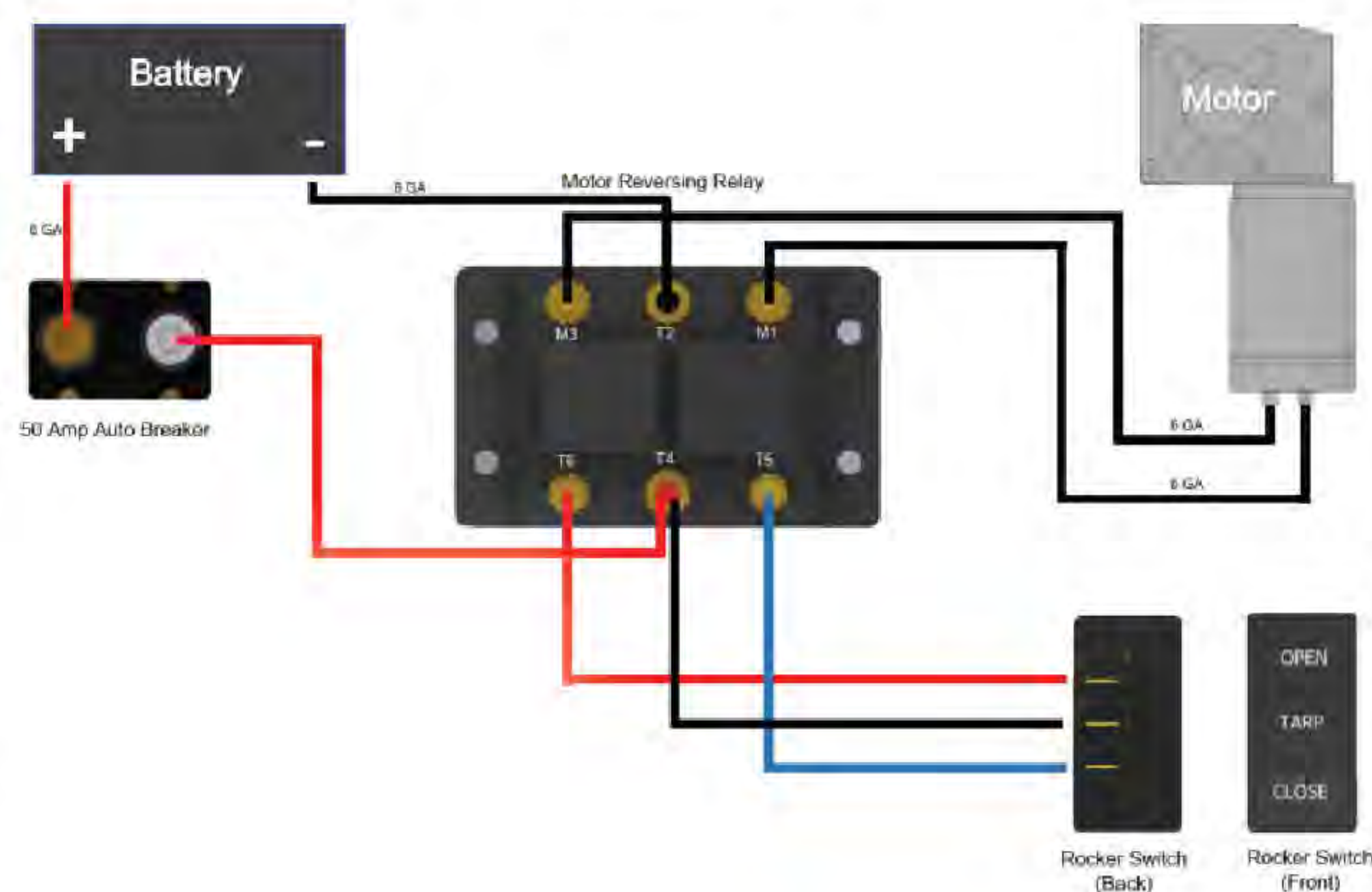
Wiring Diagram:
